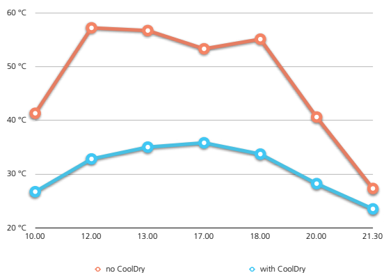
Graphique C: Béton (non-traité)
